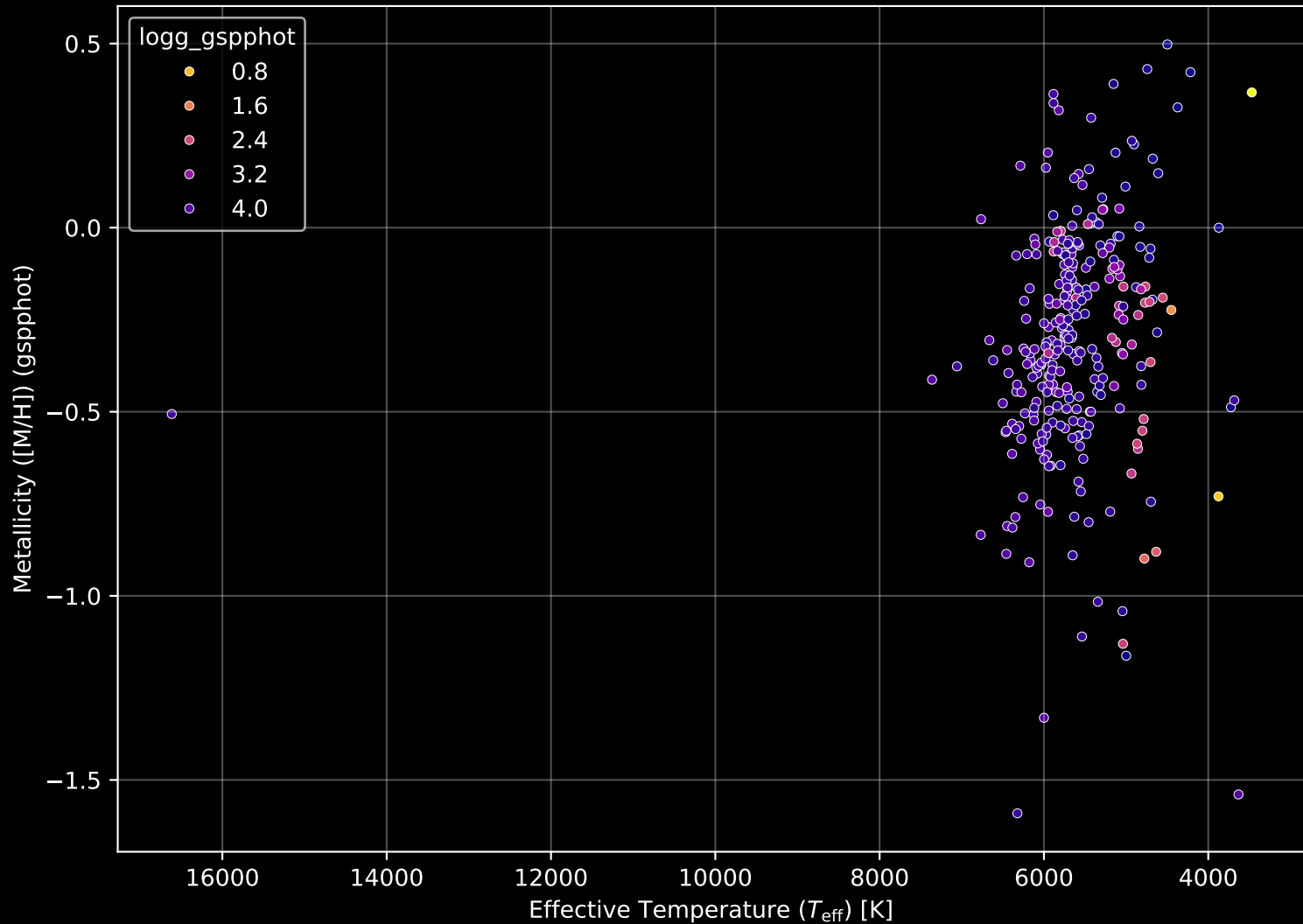
GALAH DR4 Field: [281] Stellar Population Parameters (n= 293)
