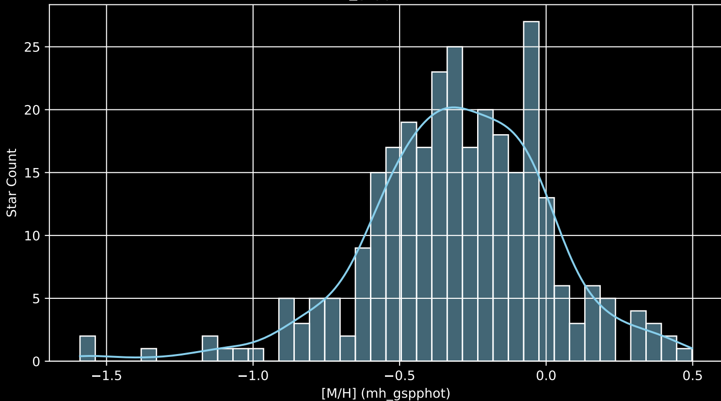
GALAH DR4 Field: [281] [M/H] (mh_gspphot) (n= 293)
