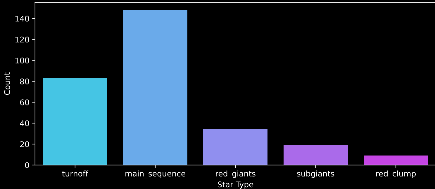
GALAH DR4 Field: [281] Count plot of Star Type
