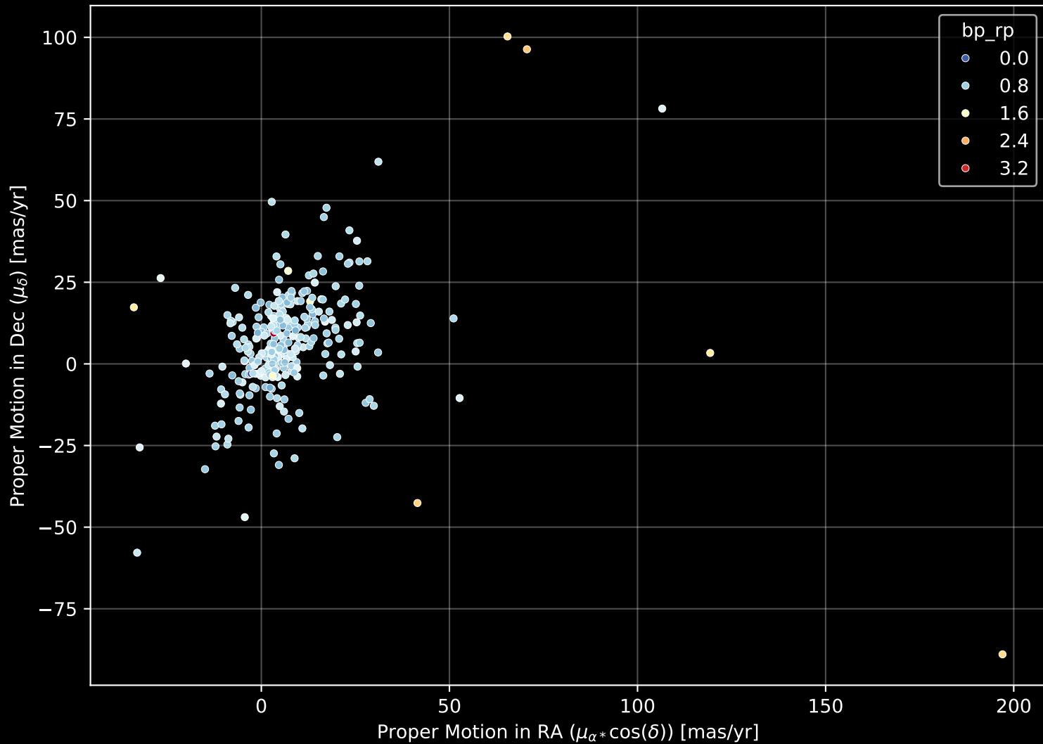
GALAH DR4 Field: [281] Proper Motion Diagram (n= 293)
