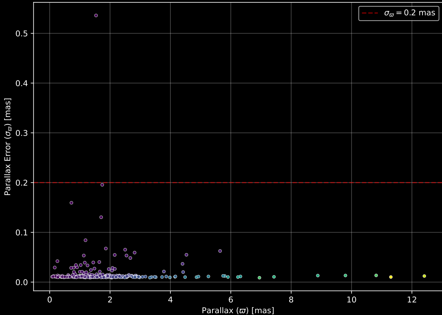
GALAH DR4 Field: [281] Parallax Quality (n= 293)
